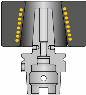
Schrumpffutter erwärmen. Heat up shrink fit chuck.
