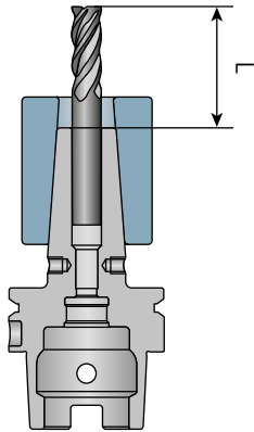
Futter vollständig abkühlen lassen mit Kühlkörper. Cool down chuck completely with cooling body.
