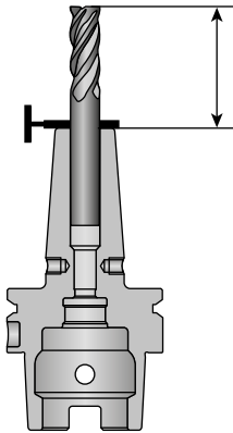
Werkzeug auf Anschlag einführen. Futter abkühlen lassen bis Werkzeug gespannt wird. Insert tool until stop. Let chuck cool down until tool is clamped.
